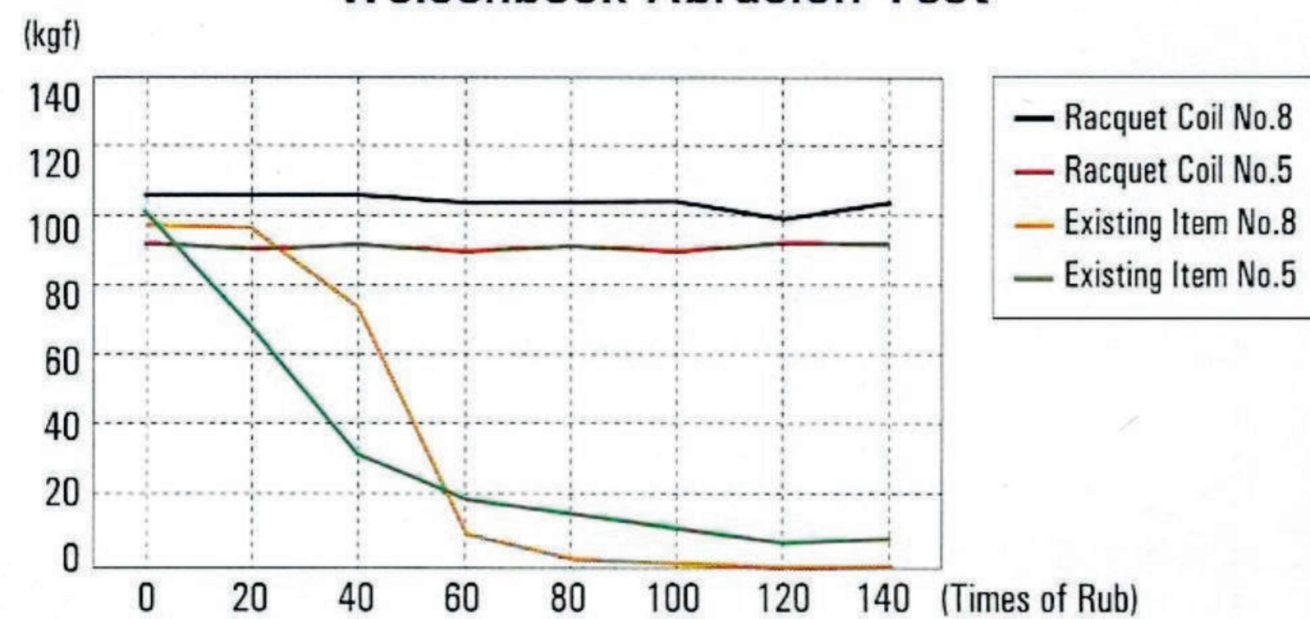
Weisenbeck Abrasion Test*
